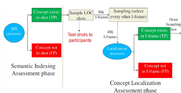
Fig. 10 2015 Evaluation Framework
