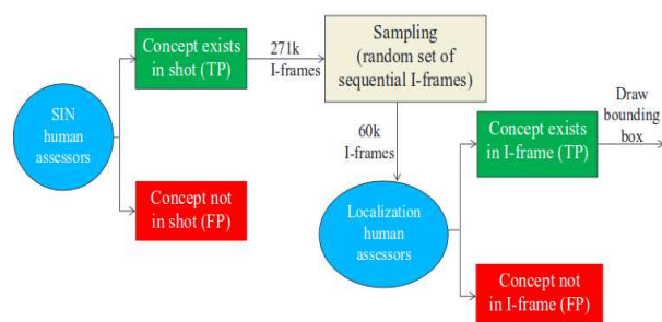
Fig. 9 2013-2014 Evaluation Framework
